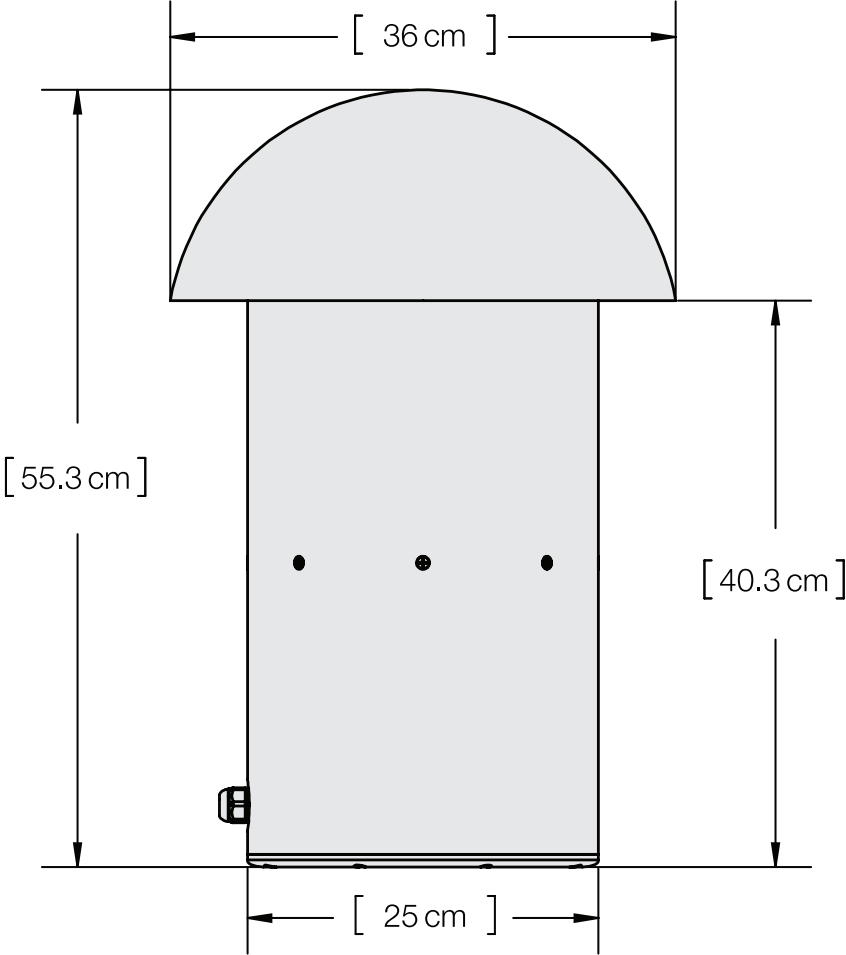
BOČNI POGLED
