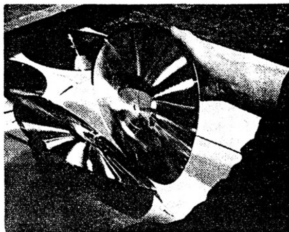
Prvi negativ »master«, srebrni s lica, odljepljuje se od niklane matrice »majke«.
